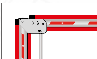
Articulation pour lisse carrée
